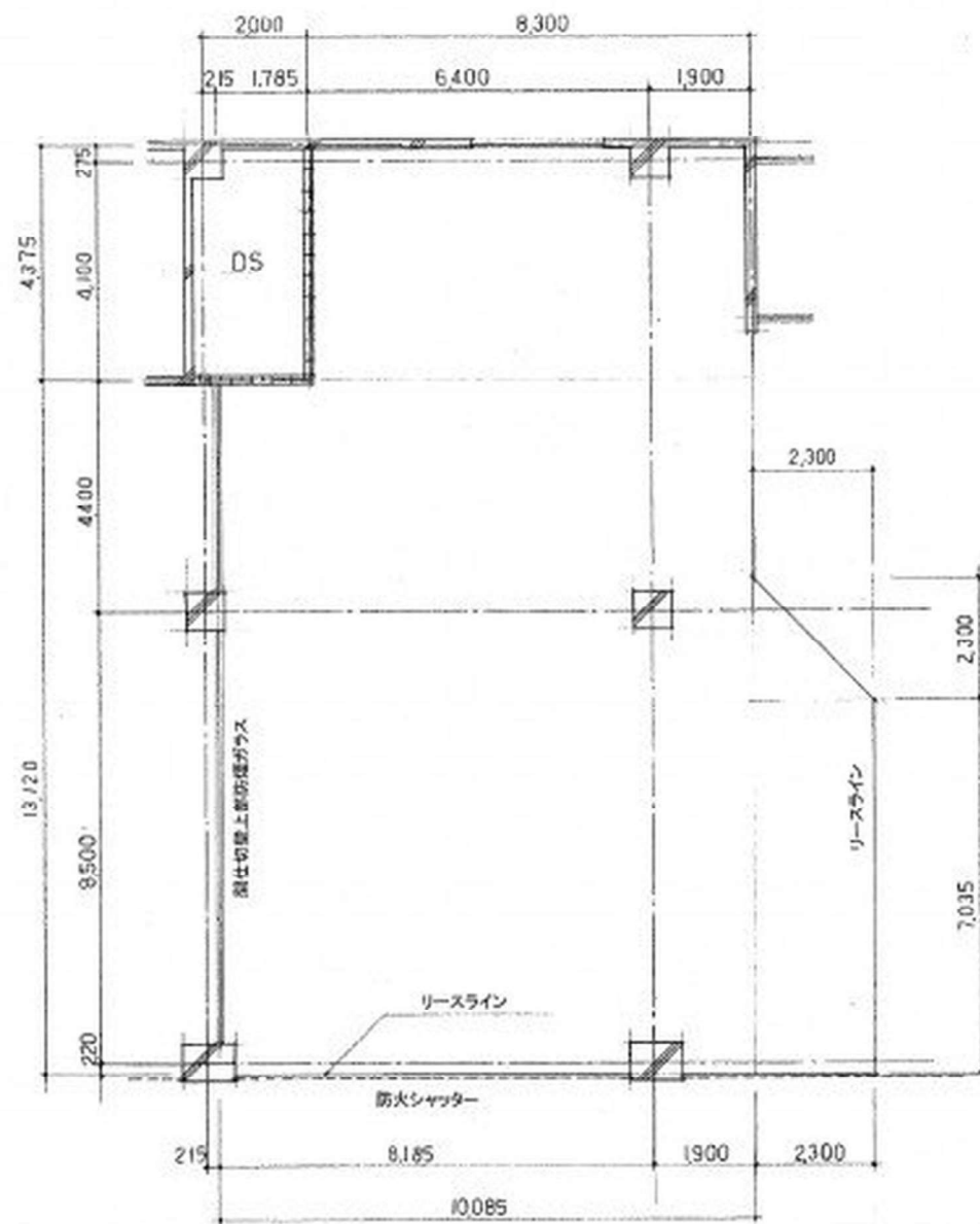
平面図 S:1/100
